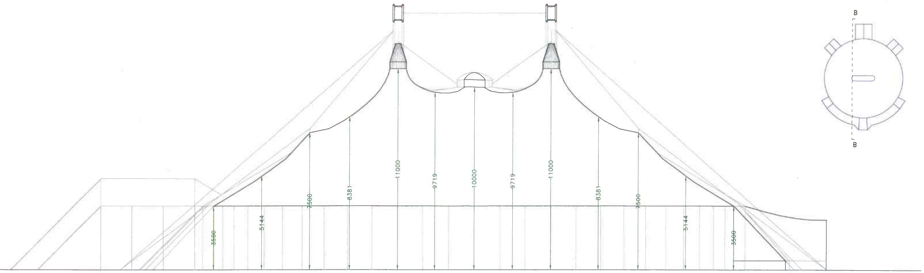
SEZIONE B-B
