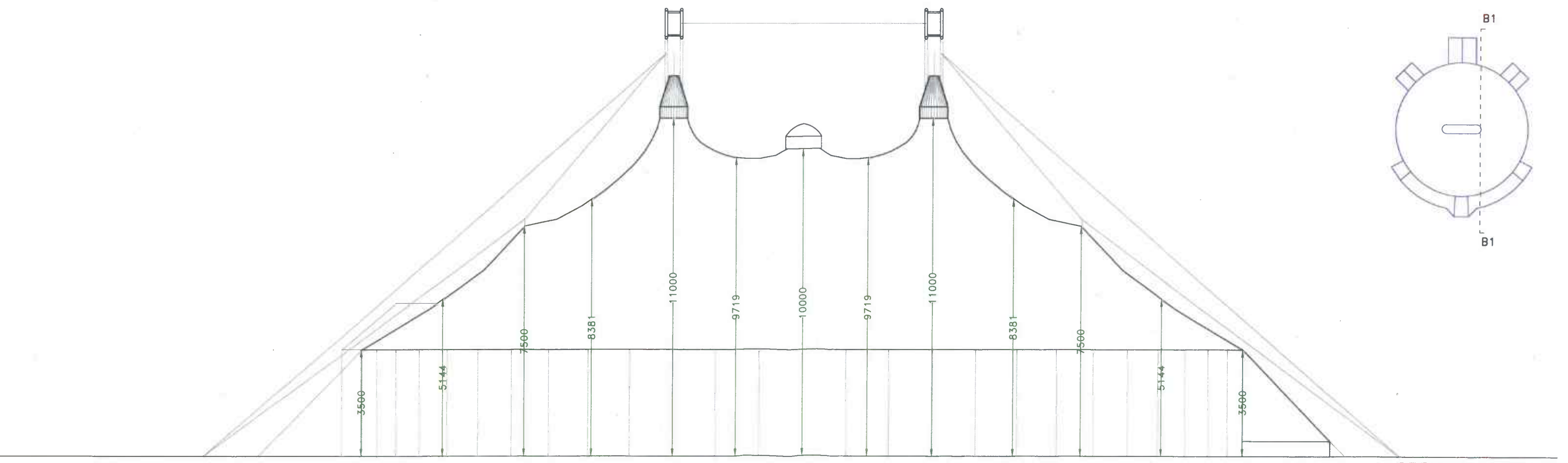
SEZIONE B1-B1
